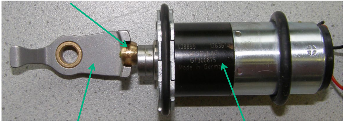
GT300880 Schwinghebel
