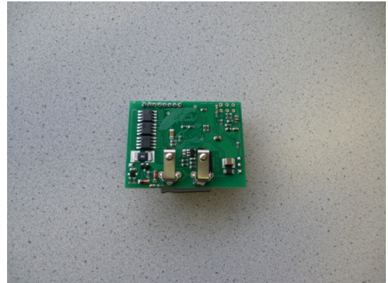
GT800855 Steuerung
