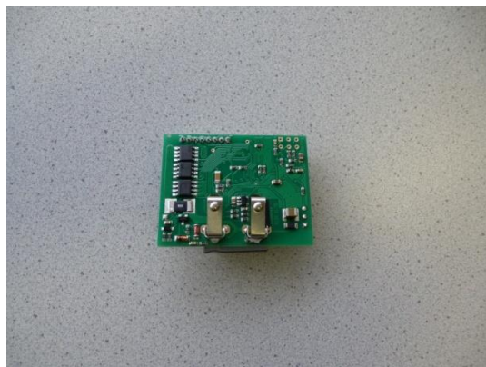
GT830850 CIRCUIT IMPRIMÉ (AVANT 03.20) GT834850 CIRCUIT IMPRIMÉ (APRES 03.20)
