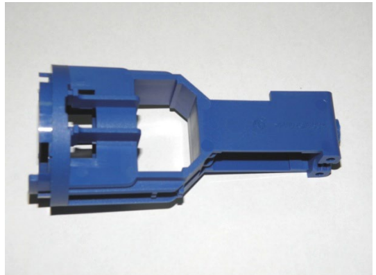
GT474842 Lagerschale
